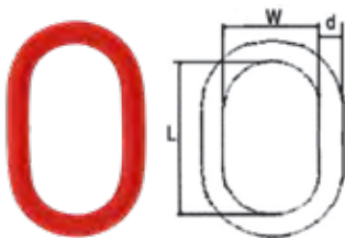
1 Aufhängeglied
